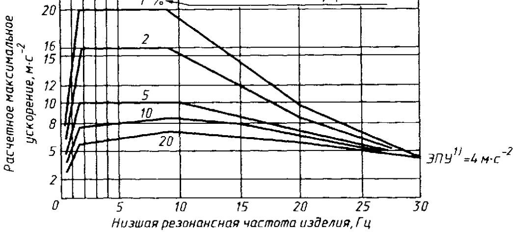
Рисунок 2 – Обобщенные спектры ответа (горизонтальное направление, 9 баллов по MSK – 64 [1])
